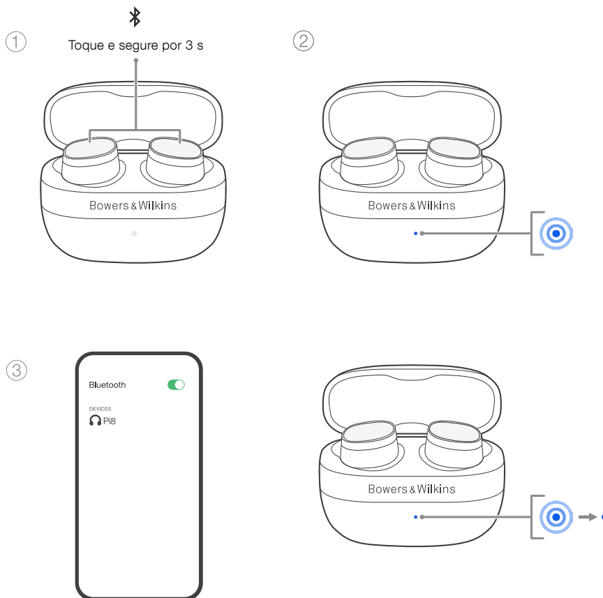
Imagem 4 Emparelhamento Bluetooth
